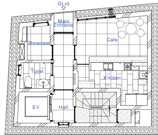
1F Plan 1:125
