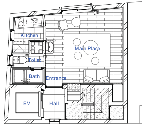
5F Plan 1:125
