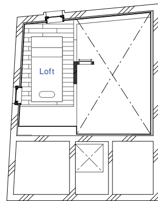
Loft Plan 1:125
