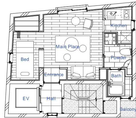
2F Plan 1:125 (3・4Fは類似したプランの為、省略。)
