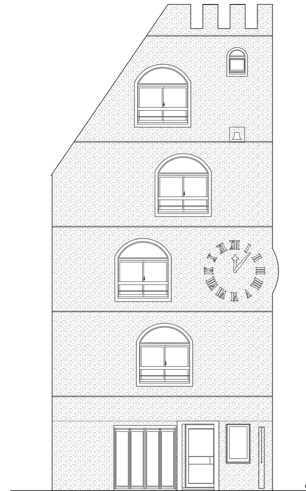
Elevation 1:125
